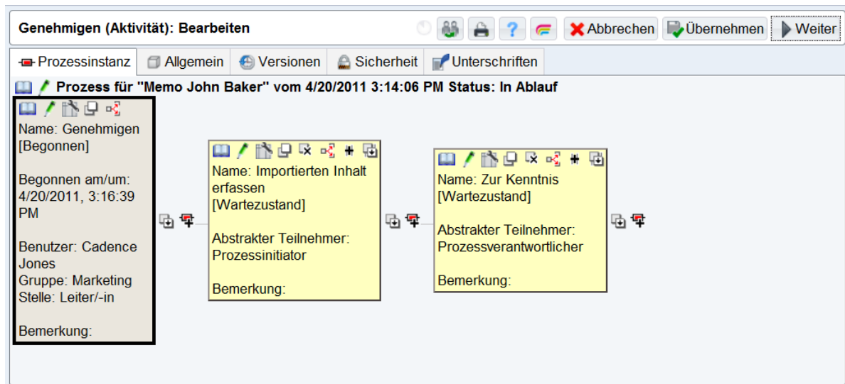
Abbildung 13: Festlegen eines Workflow Ablaufs (Ad-hoc-Workflow)
